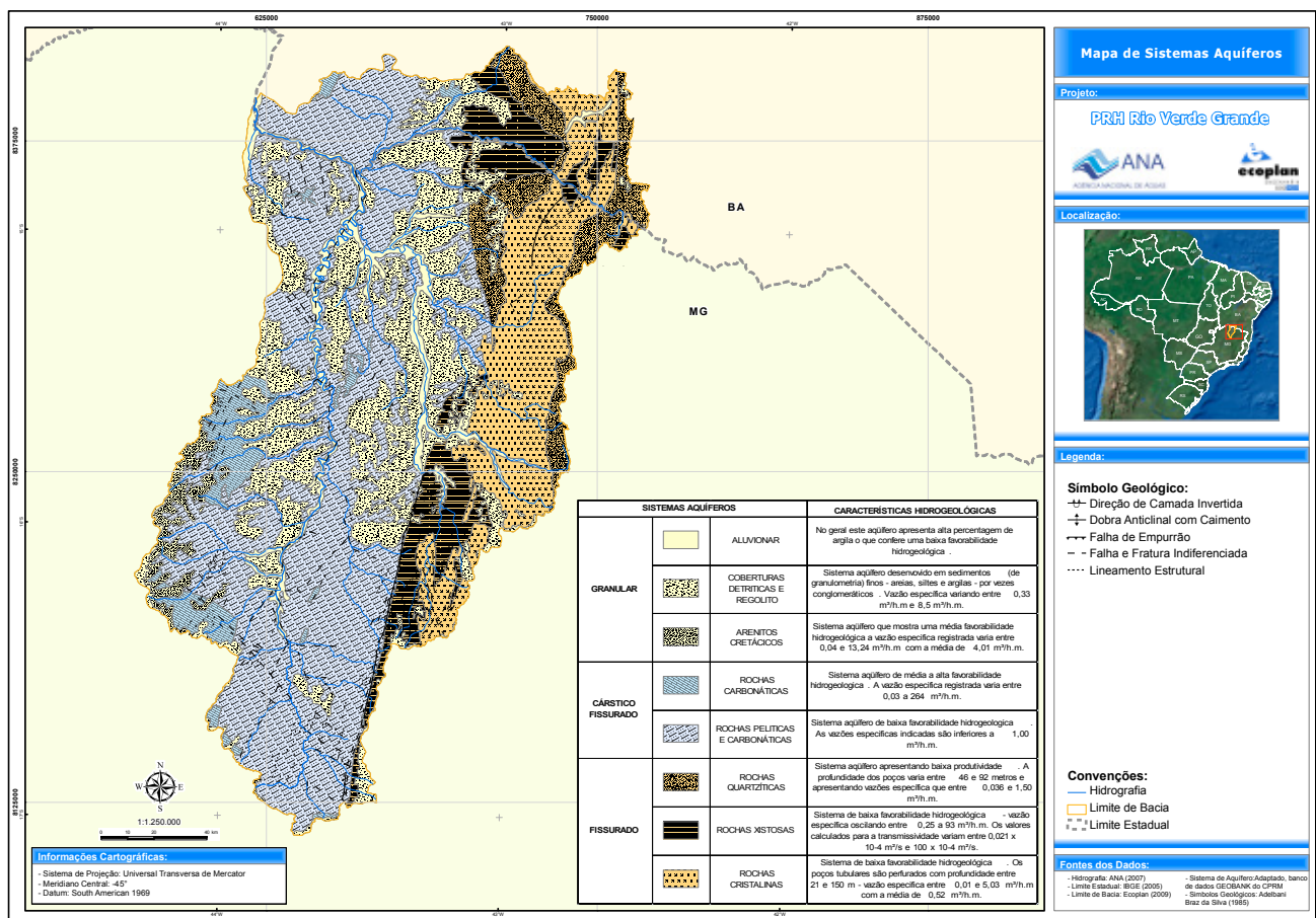
Figura 5.14 – Mapa hidrogeológico
